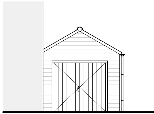
voorgevel
