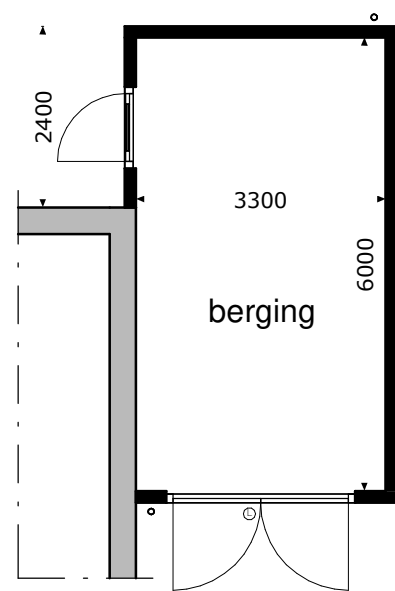
begane grond
